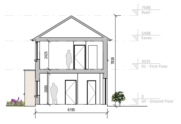
⑩ H03 Section 1 : 200
