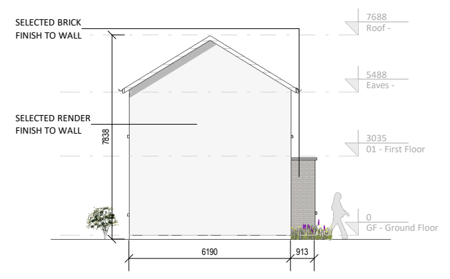
⑨ H03 Left Elevation 1 : 200
